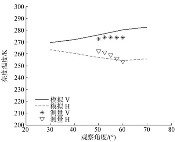
图 5 频率为 6.925 GHz 时模拟和实测的亮度温度比较(玉米)
